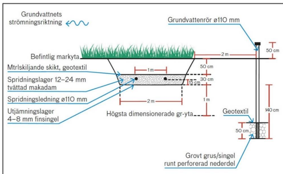
Figur 1. Exempel på tvärsnittsritning över infiltration med grundvattenrör för kontroll av grundvattennivå. Rörets botten bör ligga minst 140 cm under infiltrationsnivån (undre kanten på spridningslagret i detta exempel). Bifoga en tvärsnittsritning som underlag för installationsarbetet till din ansökan.
