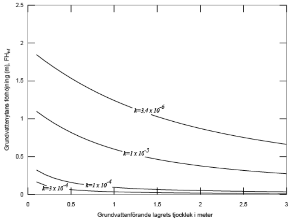
Figur 5. Grundvattennivåns förhöjning ( FH_{inf} ) som funktion av grundvattenförande lagrets tjocklek vid några olika k -värden. Kurvorna är beräknade baserat på metod beskriven av Finnemore 1993 2 .
